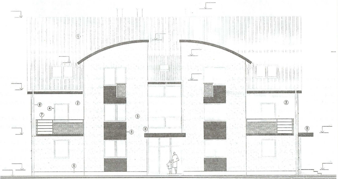
Pohľad západný
